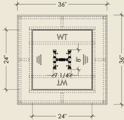
TOP ELEVATION
